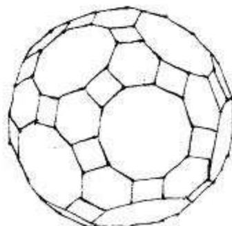
ICOSI-DODECAEDRE TRONQUE
