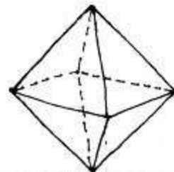
OCTAÈDRE
